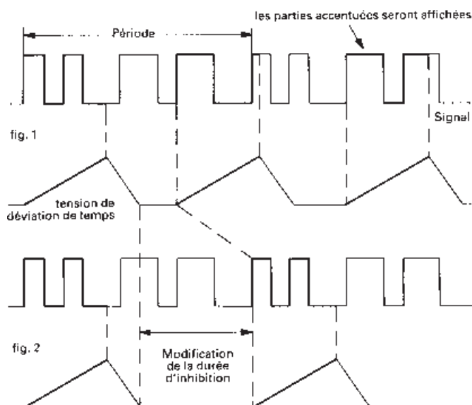
La fig. 1 montre l'écran avec le bouton de réglage HOLD-OFF en butée à gauche (position de base). Étant donné que différentes parties de la courbe sont affichées, il n'y a pas d'image fixe représentée (écriture double).
